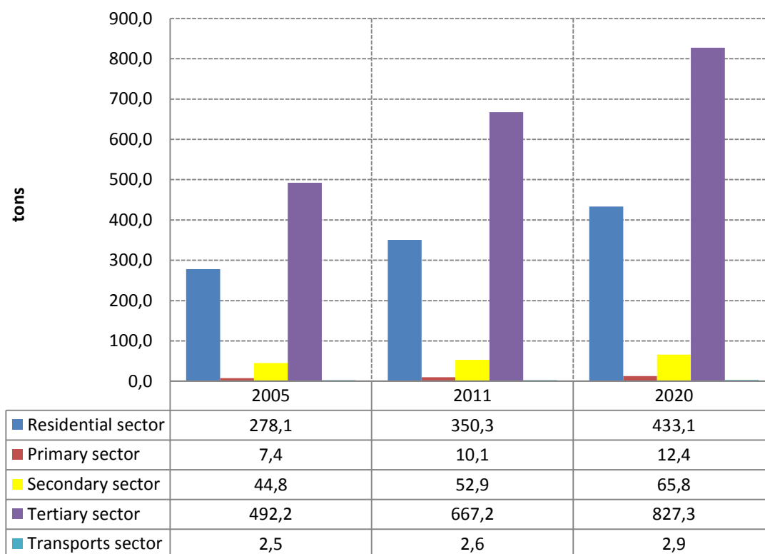
Διάγραμμα 3.28. BAU σενάριο – Προβολή εκπομπών CO 2 τελικής χρήσης ανά ενεργειακό φορέα
