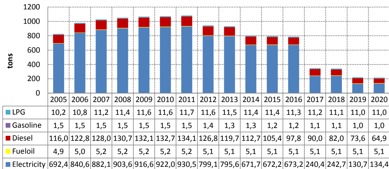
Διάγραμμα 3.39. ΝΣΔΑΕ σενάριο – Προβολή εκπομπών CO 2 τελικής χρήσης ανά ενεργειακό φορέα
