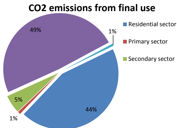
Διάγραμμα 3.13. Κατανομή συνολικών εκπομπών CO 2 από τελική χρήση στους διάφορους τομείς
