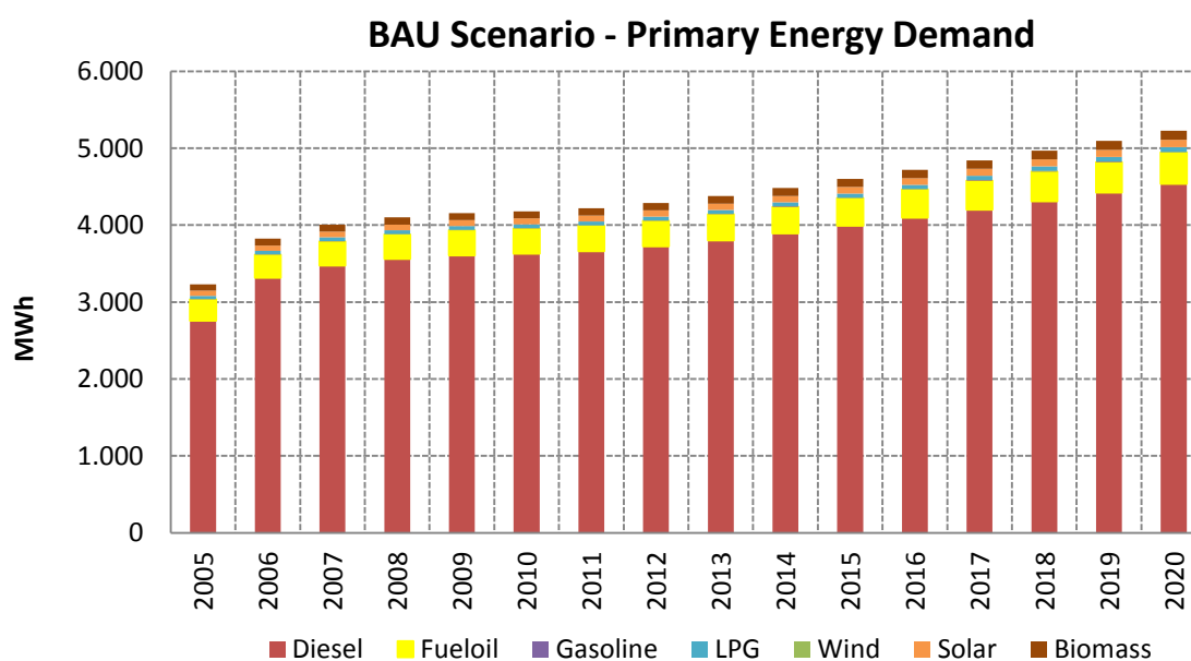
Διάγραμμα 3.24. BAU σενάριο – Προβολή πρωτογενούς ζήτησης ενέργειας ανά ενεργειακό φορέα
